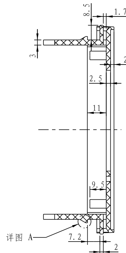
剖面 A-A
