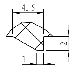
细节 A 比例 3:1
