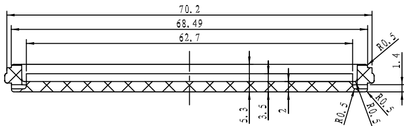
剖面 P-P
