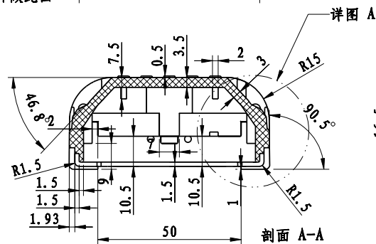
剖面 A-A
