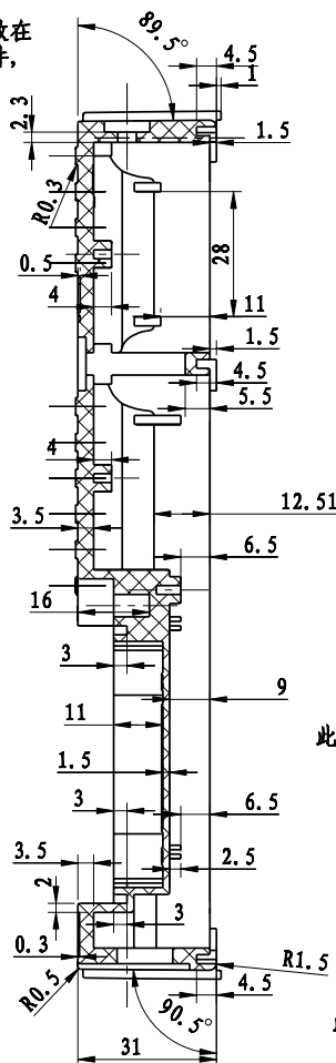
剖面 B-B
